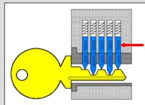
Sezione longitudinale di una serratura Pin Tumbler.
