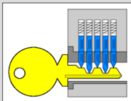
Sezione longitudinale di una serratura Pin Tumbler.
