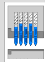
Sezione longitudinale di una serratura Pin Tumbler.
