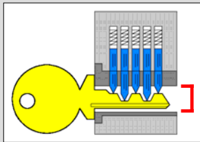
Sezione longitudinale di una serratura Pin Tumbler.
